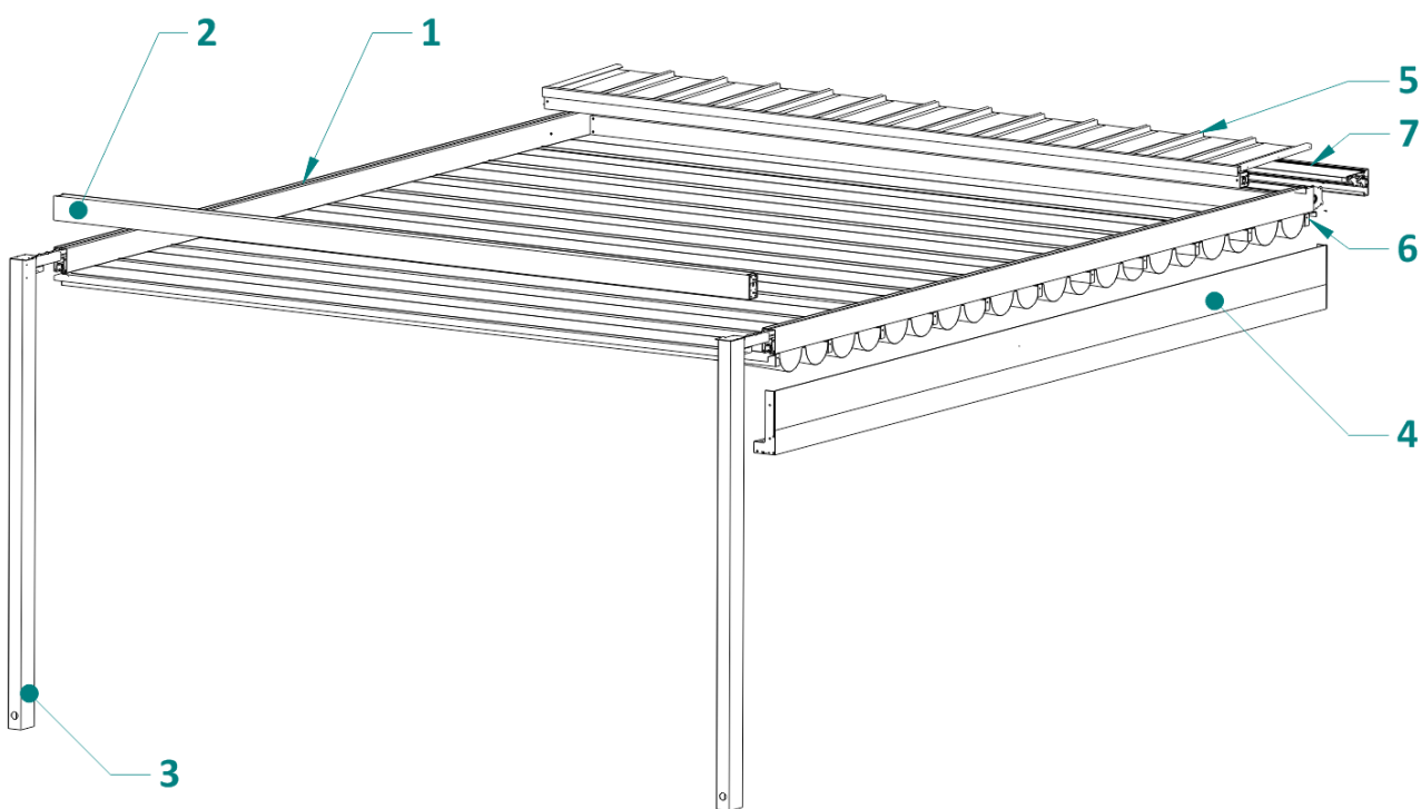
Rys. 3.1b Graficzne przedstawienie konstrukcji przyściennej Tarasola FLAT.
