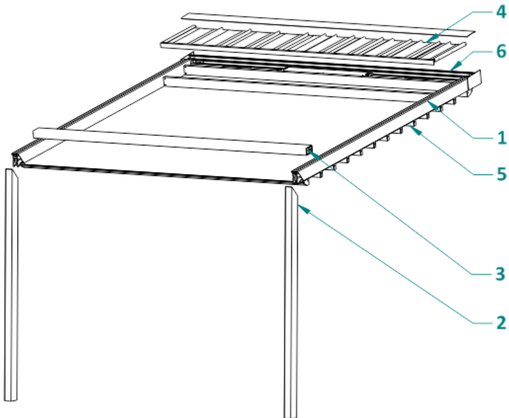
Rys. 3.1a Graficzne przedstawienie konstrukcji Tarasola LIGHT z dodatkowym profilem spinającym.
