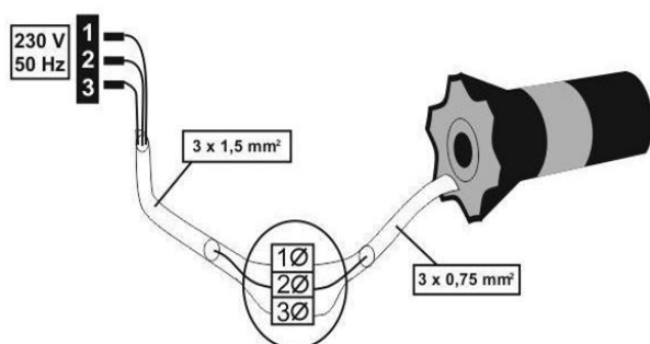
Rys. 3 Napęd elektryczny ze zdalnym sterowaniem.
