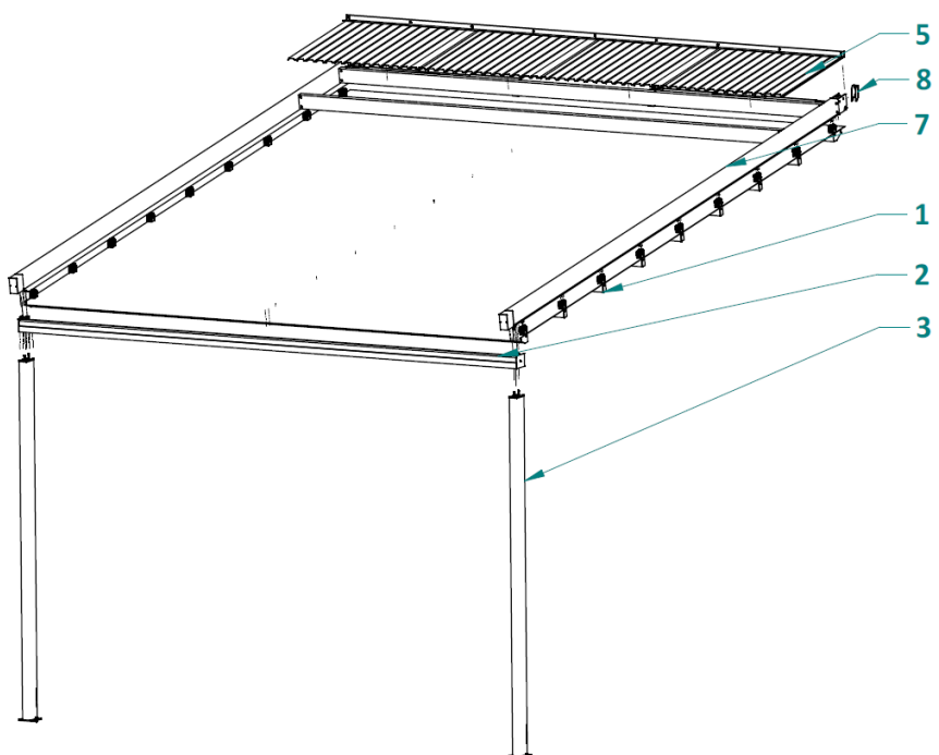
Rys. 2 Graficzne przedstawienie konstrukcji Simple z napędem elektrycznym
