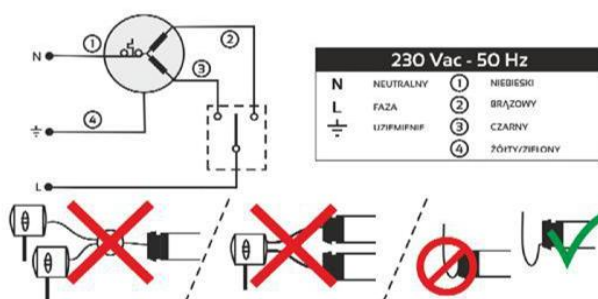
Rys. 4 Napęd elektryczny z włącznikiem.
