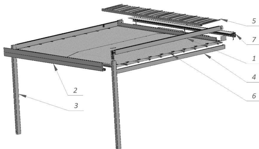
Rys. 2 Graficzne przedstawienie konstrukcji przyściennej Tarasola Cubic
