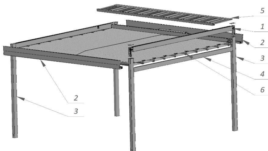
Rys. 1 Graficzne przedstawienie konstrukcji wolnostojącej Tarasola Cubic
