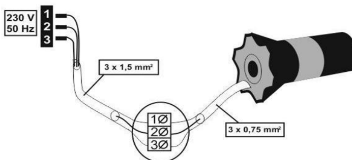
Rys. 4 Napęd elektryczny ze zdalnym sterowaniem
