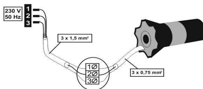
Rys. 3 Napęd elektryczny ze zdalnym sterowaniem.
