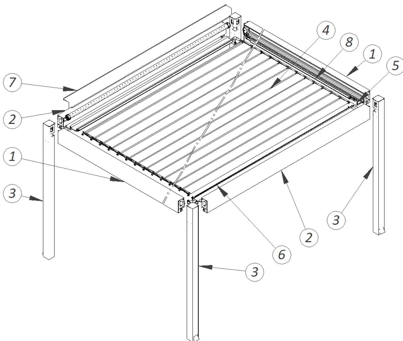
Rys.1 Graficzne przedstawienie konstrukcji Tarasola Technic View
