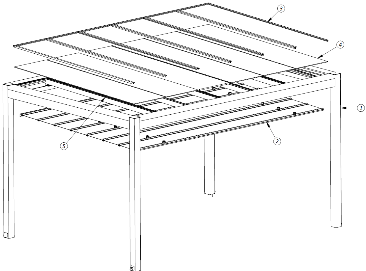
Rys.2 Graficzne przedstawienie konstrukcji Tarasola Technic w wersji z dachem szklanym
