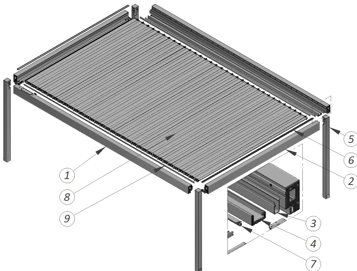
Rys.1 Graficzne przedstawienie konstrukcji Tarasola Technic
