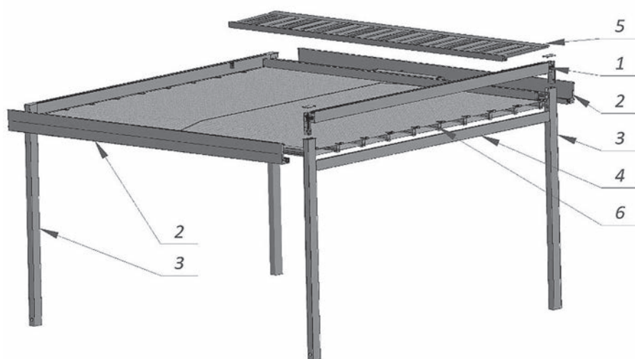
Rys.1 Graficzne przedstawienie konstrukcji wolnostojącej Tarasola Cubic
