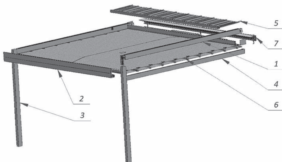
Rys.2 Graficzne przedstawienie konstrukcji przyściennej Tarasola Cubic
