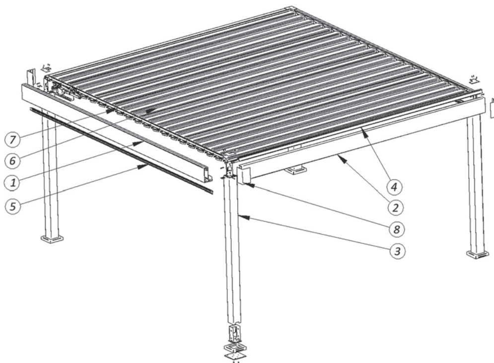
Rys.1 Graficzne przedstawienie konstrukcji Tarasola Essential
