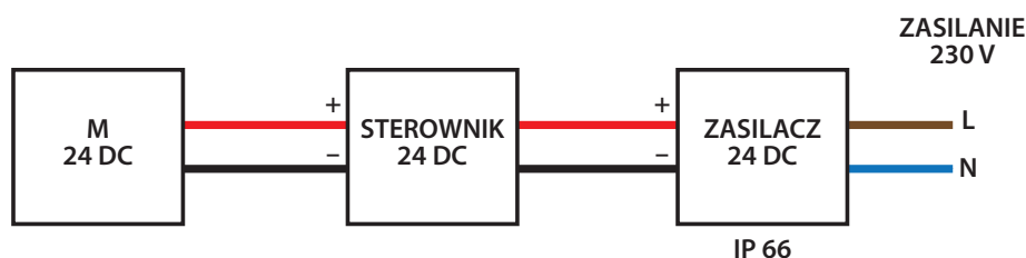
Rys.2 Schemat podłączenia silnika
