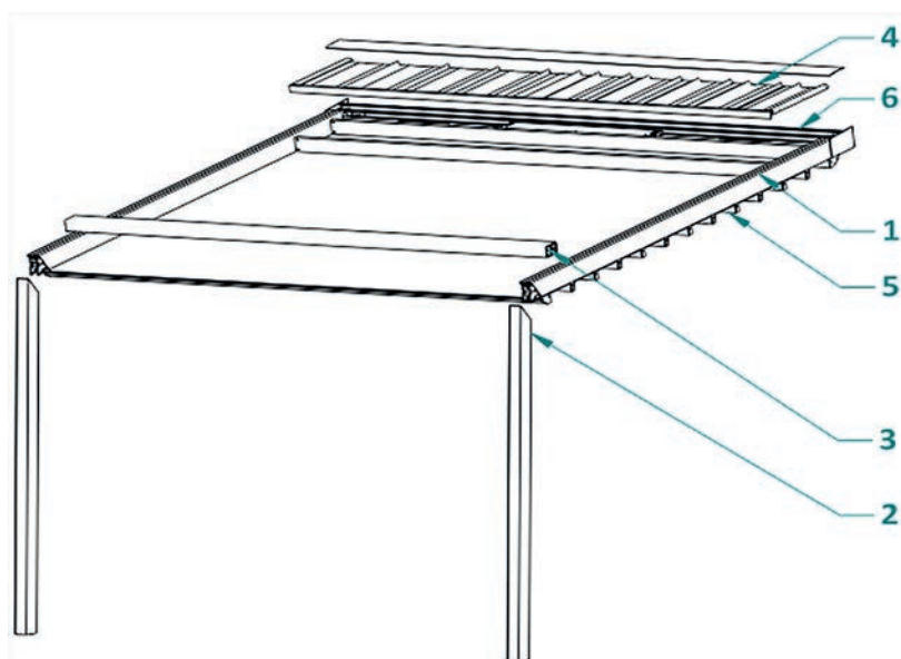
Rys. 2 Graficzne przedstawienie konstrukcji Tarasola Light z dodatkowym profilem spinającym.
