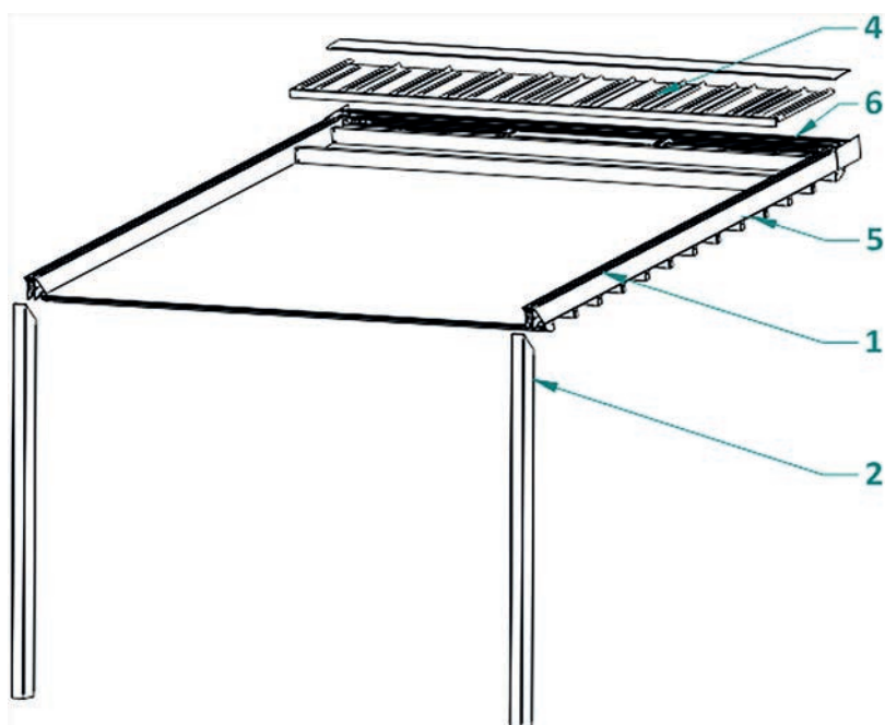
Rys. 1 Graficzne przedstawienie konstrukcji Tarasola Light
