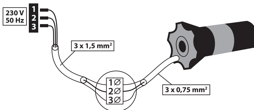
Rys. 4 Napęd elektryczny ze zdalnym sterowaniem.
