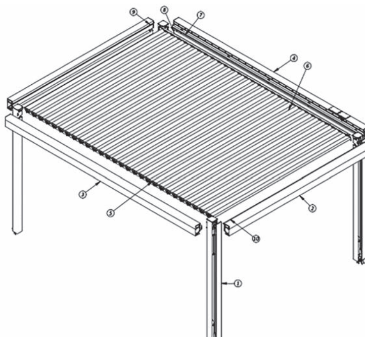
Rys. 1 Graficzne przedstawienie konstrukcji Tarasola Technic Pro
