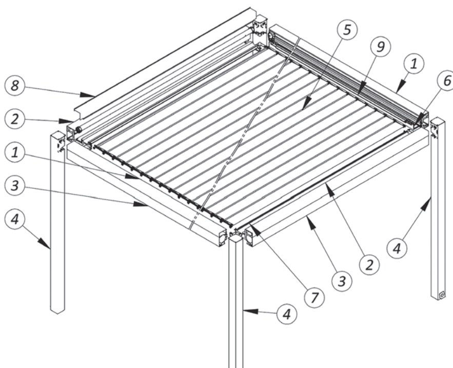
Rys.1 Graficzne przedstawienie konstrukcji Tarasola Technic View Pro
