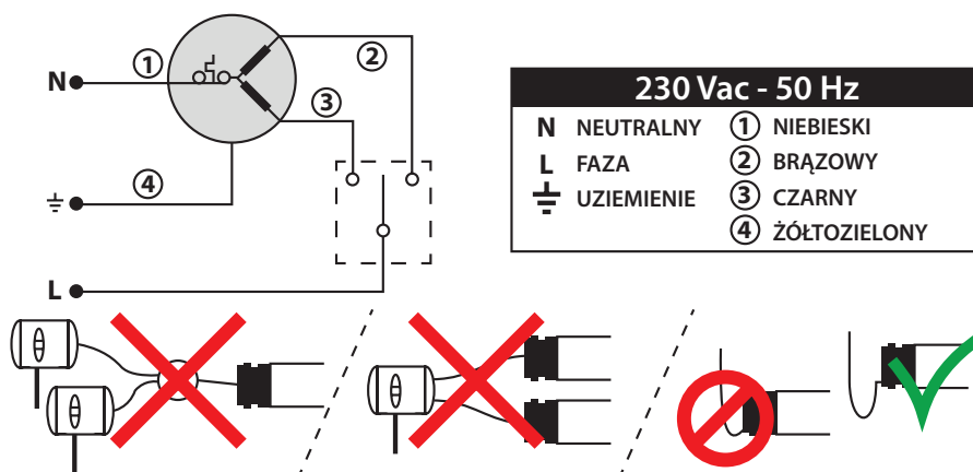
Rys. 3 Napęd elektryczny z włącznikiem.
