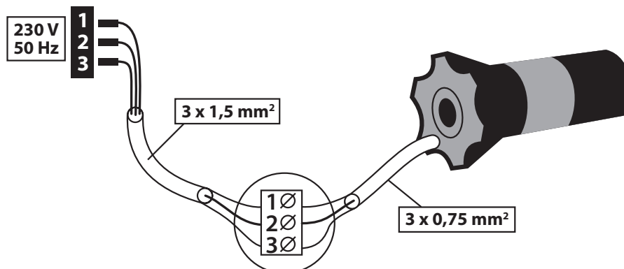
Rys. 2 Napęd elektryczny ze zdalnym sterowaniem
