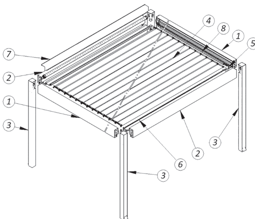
Rys.1 Graficzne przedstawienie konstrukcji Tarasola Technic View
